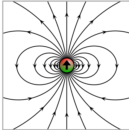
Fig. 2. – Dipole magnétique
